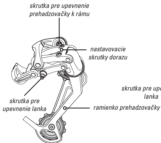
obrázok 23 - popis prehadzovačky
