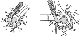
obrázok 10 - umiestnenie rýchloupínačov
