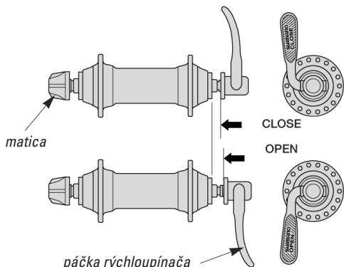
obrázok 7 - pozícia rýchloupínača
